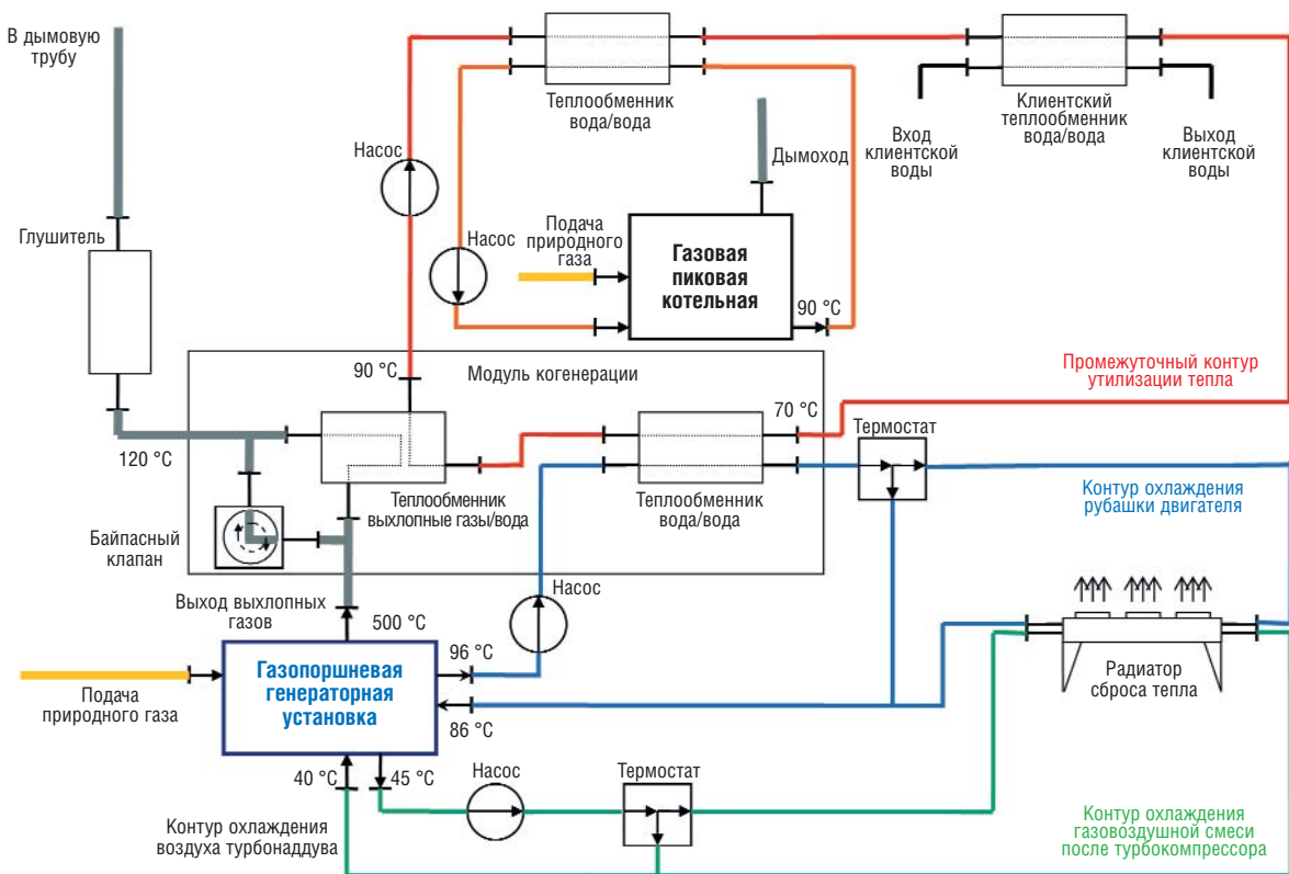
Рис. Структурная схема системы утилизации тепла для оборудования FG Wilson
